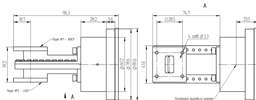
Рисунок 1 – Общий вид изделия.
